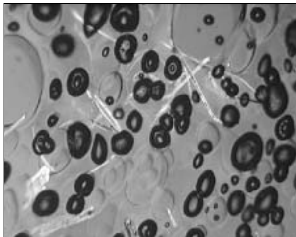
■ 3. ÁBRA. Poliuretán hulladékból előállított lencsával erősített, zárt cellás hab mikroszkópi képe
